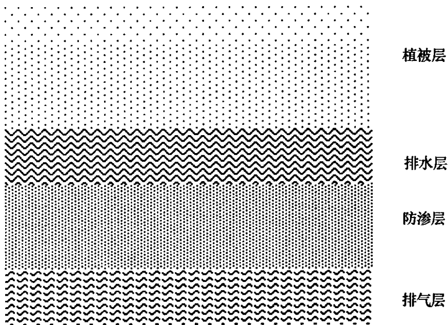
图 5.0.2 封场覆盖系统结构示意图
